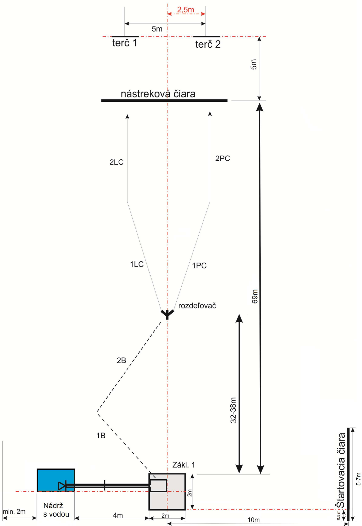
Príloha č. 1: - Grafický plánik s rozmermi súťažnej trate:
